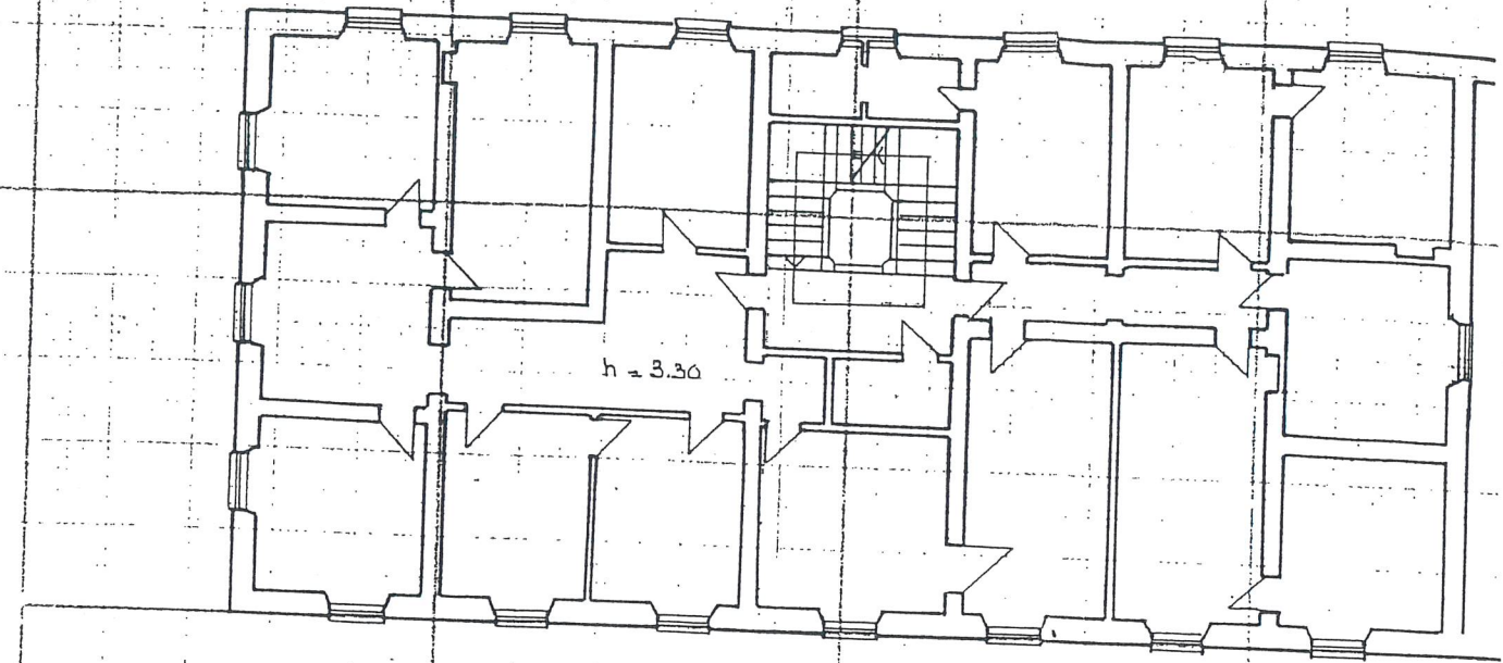
PIANO PRIMO
