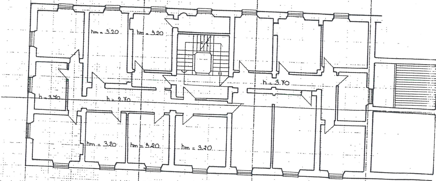
PIANO SECONDO
