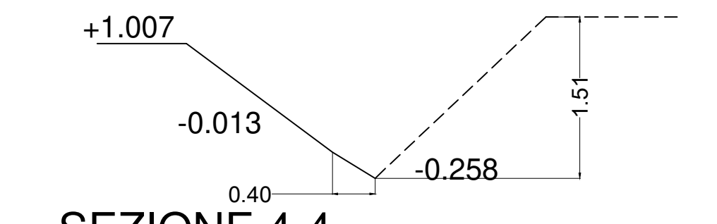
SEZIONE 4-4
