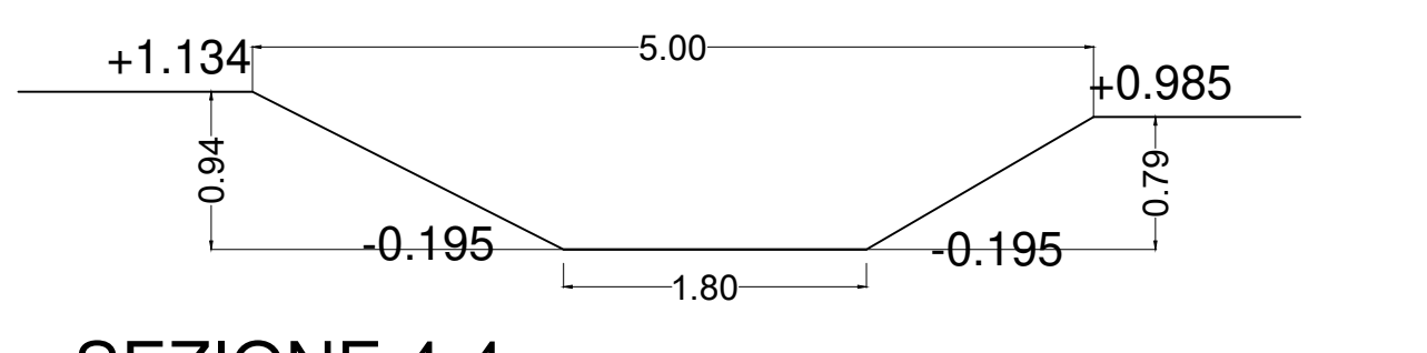
SEZIONE 4-4
