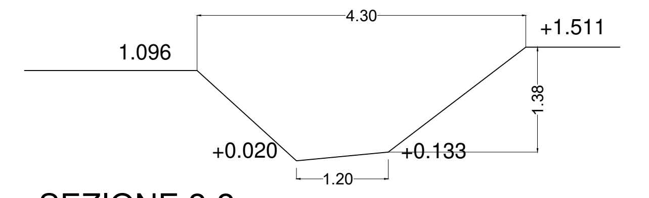
SEZIONE 2-2
