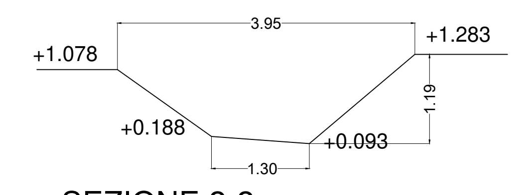
SEZIONE 2-2
