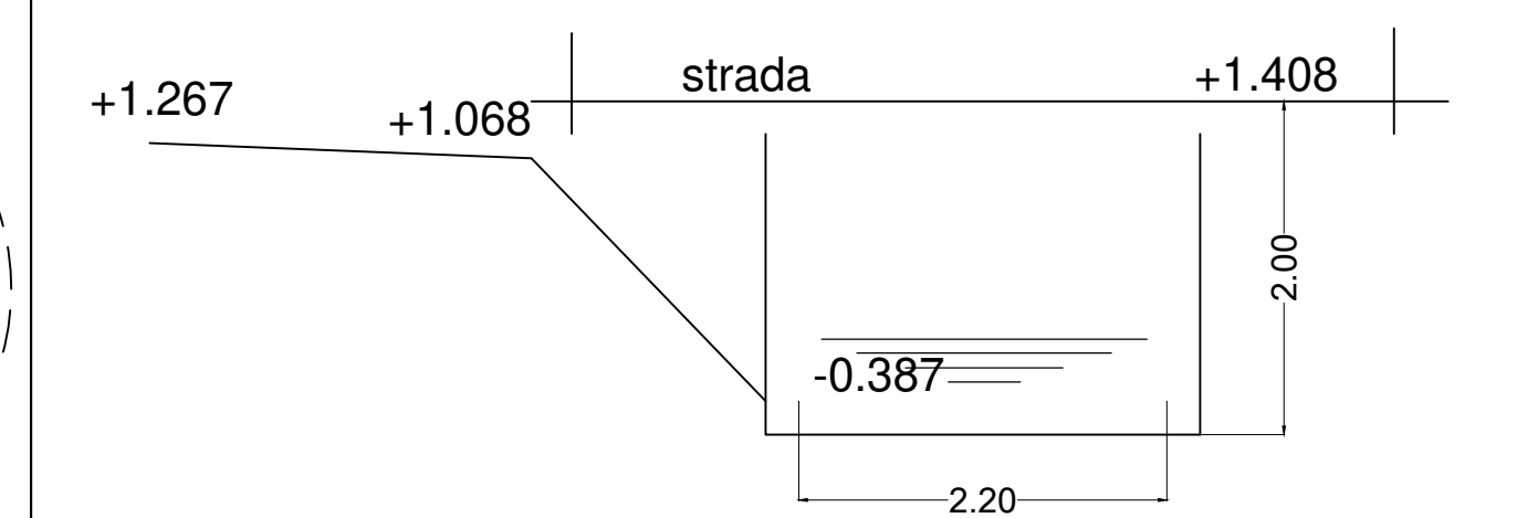
SEZIONE 3-3
