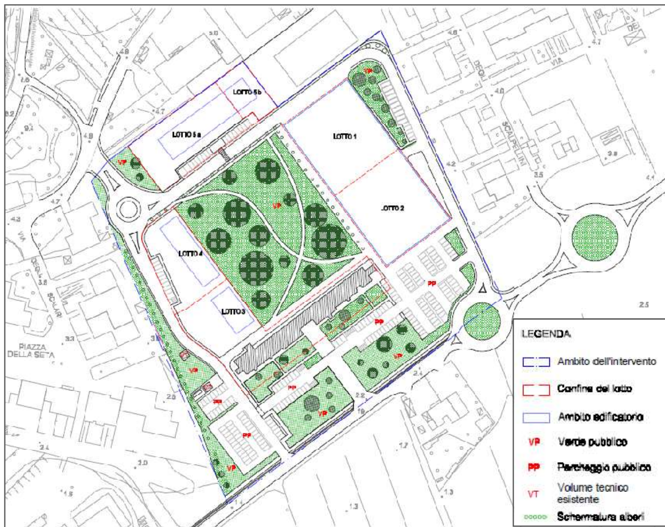
Estratto Tav. 4 - Soluzione progettuale in variante modificata a seguito dell'accoglimento delle osservazioni
